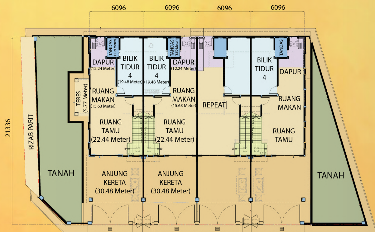
PELAN LANTAI ARAS BAWAH
